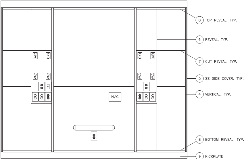
SECTION-A
